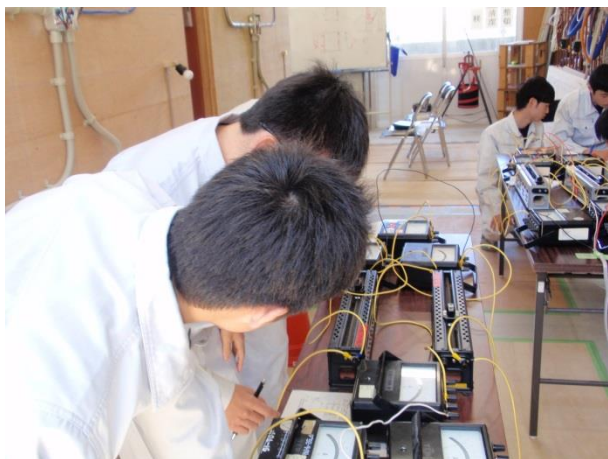
単相三線式の実験
